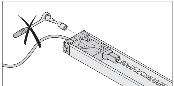
Abb. 8. Einschubteil mit Steuerleitung
