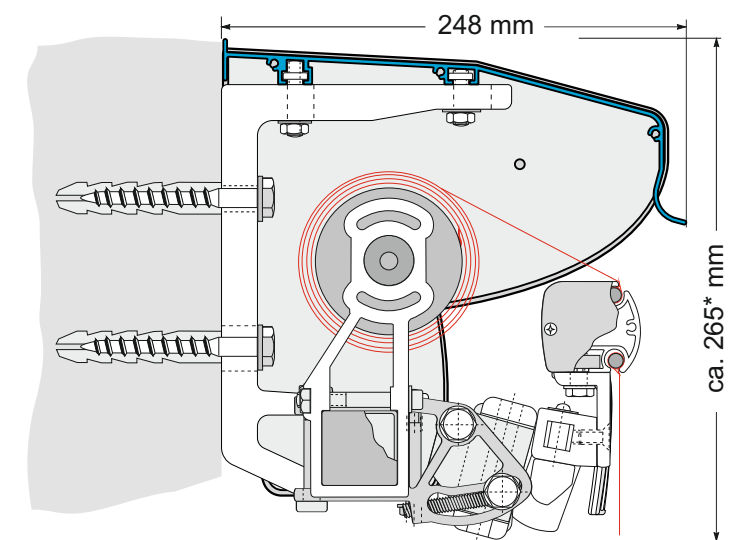
Wandmontage mit Regenschutzdach Wall mounting with rain cover
