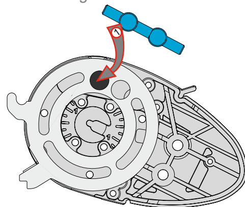
Einhängung in Einschnitt / Fitting in recess 1
