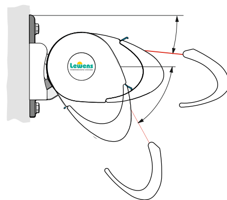
Motorbedienung / Motor control 5°-65° Handbedienung / Hand control 5°-55°
