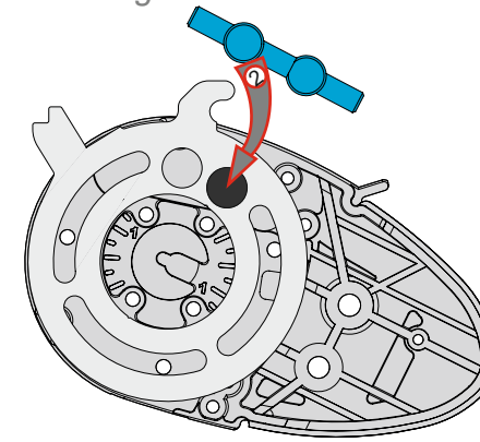
Einhängung in Einschnitt / Fitting in recess 2
