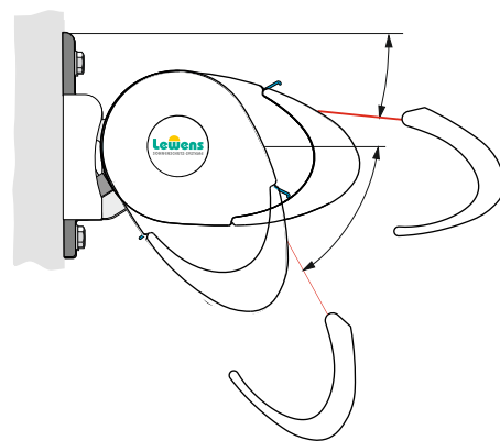
Motorbedienung / Motor control 20°-80° Handbedienung / Hand control 20°-55°
