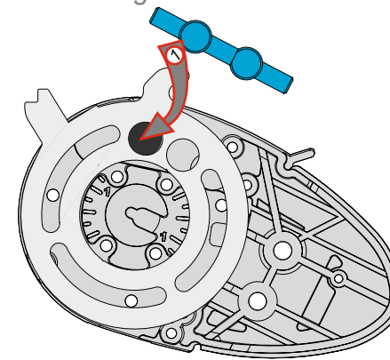
Einhängung in Einschnitt / Fitting in recess 1
