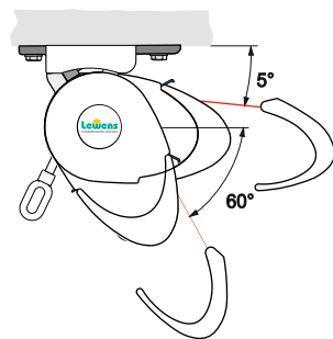
Bedienung Kurbel Operation Crank 5° - 60°
