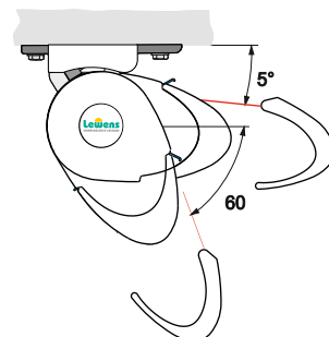
Bedienung Motor Operation Motor 5° - 60°
