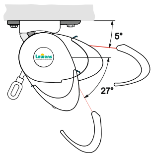
Bedienung Kurbel Operation Crank 5° - 27°
