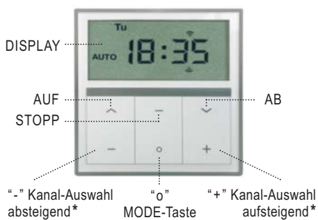
(Abb. 1) Tastenbelegung:
